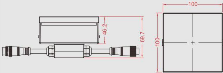
尺寸图/Size 单位: mm
