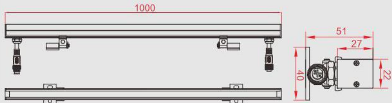
尺寸图/Size 单位: mm
