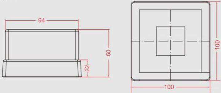
尺寸图/Size 单位: mm
