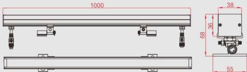
尺寸图/Size 单位: mm
